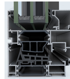
Level 1 Uf: \geq 0.28 Btu/hr.ft 2 .°F
